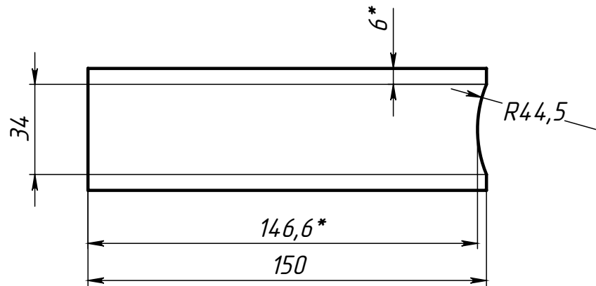
Поз.1 (Основание)
